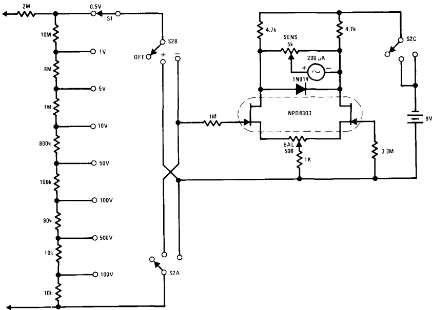
FETVM-FET Voltmeter
